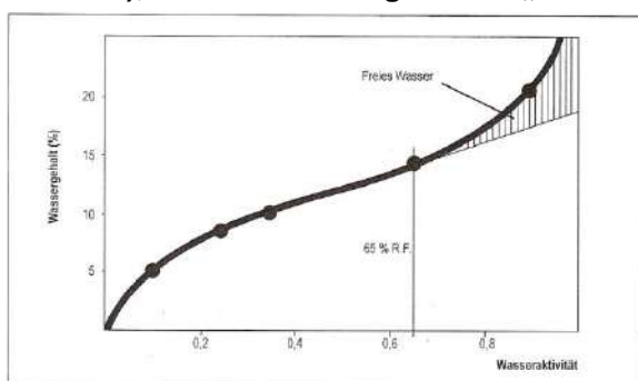
Abb. 11-8: Sorptionsisotherme von Getreide (K. Klingler)
